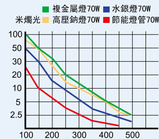
配光曲線圖
