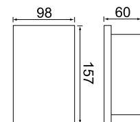
預埋盒尺寸
