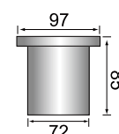
91034預埋筒尺寸
