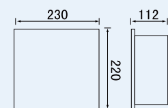
91892 91893預埋盒尺寸
