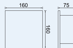
預埋盒尺寸
