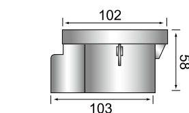
91031~91033預埋筒尺寸
